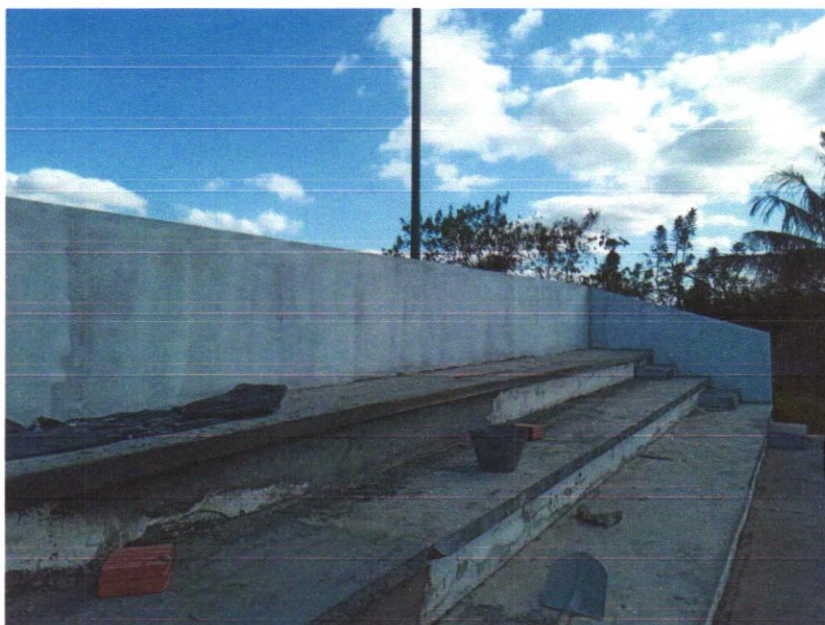
Foto 02 – MASSA ÚNICA, PARA RECEBIMENTO DE PINTURA, EM ARGAMASSA TRAÇO 1:2:8, PREPARO MANUAL, APLICADA MANUALMENTE EM FACES INTERNAS DE PAREDES, ESPESSURA DE 10MM, COM EXECUÇÃO DE TALISCAS
